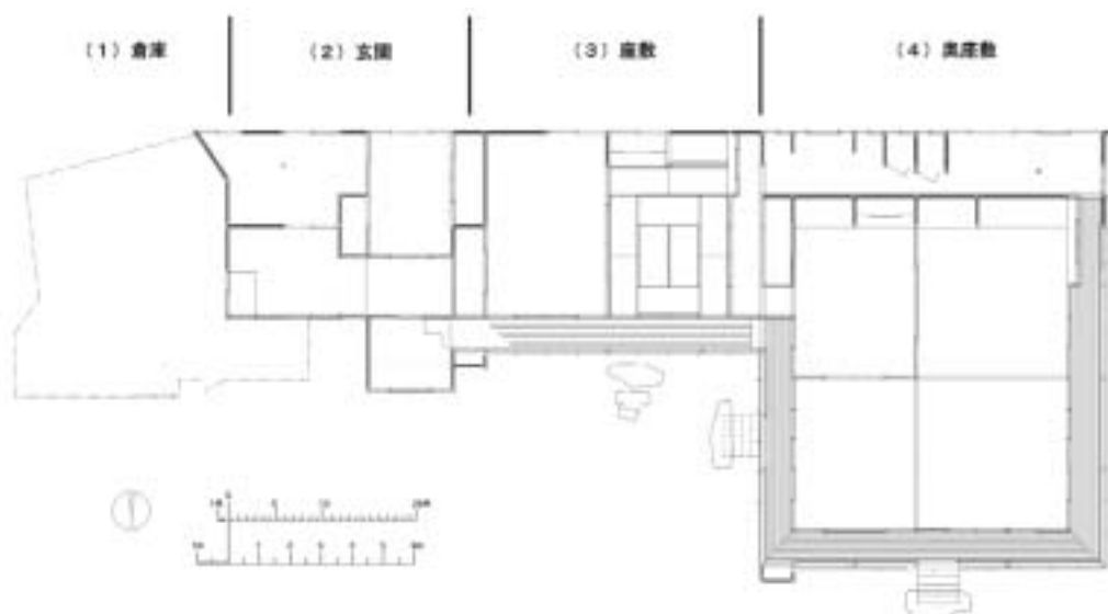
図6：「あしべ屋別荘」、略平面図（作図：西本直子）
