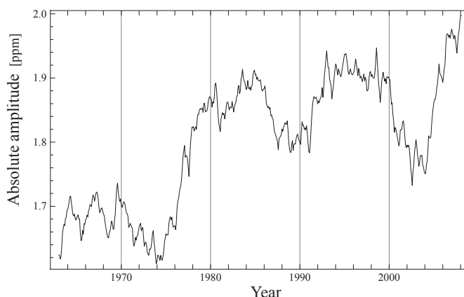
図 9 季節変動振幅の絶対値の年々変動
