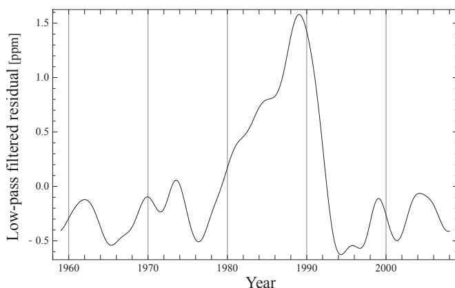
図7 ローパスフィルタにより残差から短周期変動分を取り除いた結果
