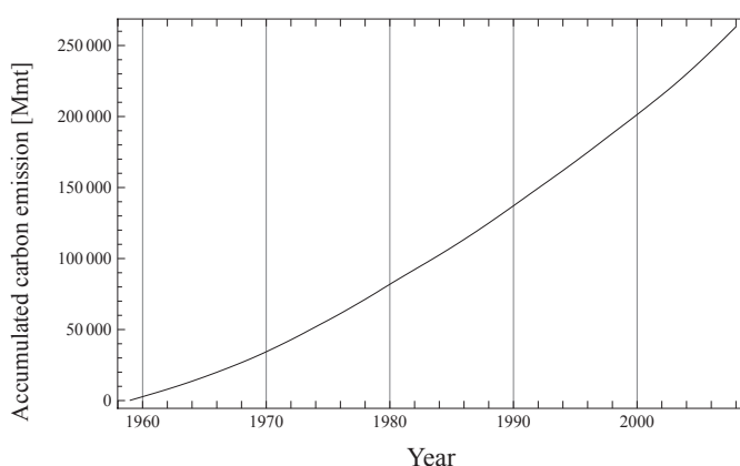
図3 排出された炭酸ガスの積算量の推移
