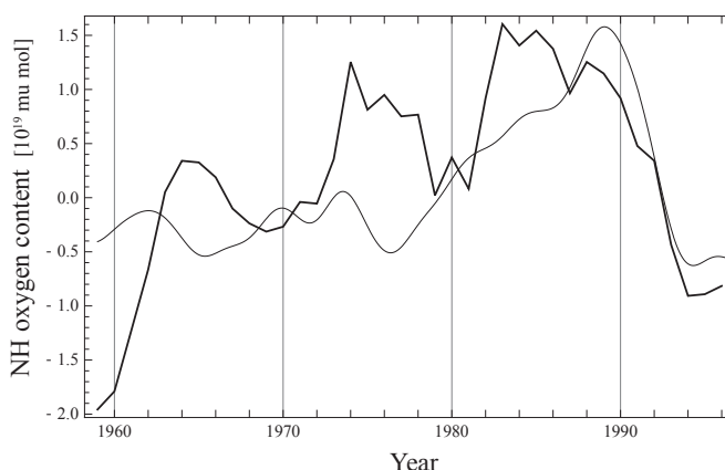
図 11 北半球海洋中の酸素濃度とスケーリングした長周期残差の比較 (太線が酸素濃度)
