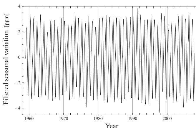
図 8 1 年程度の短周期成分を取り除いた後の季節変動振幅
