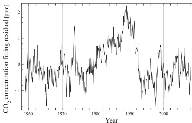
図6 大気中炭酸ガスの変動から化石燃料燃焼により排出された量の積算値と季節変動を取り除いた残差
