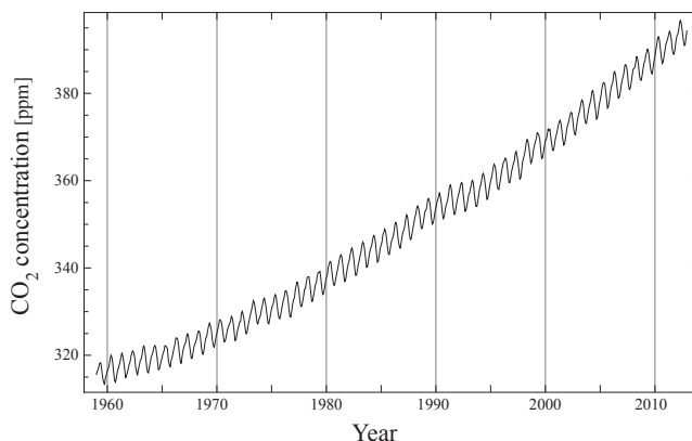
図1 Mauna Loaにおいて観測された大気中炭酸ガス濃度の変化
