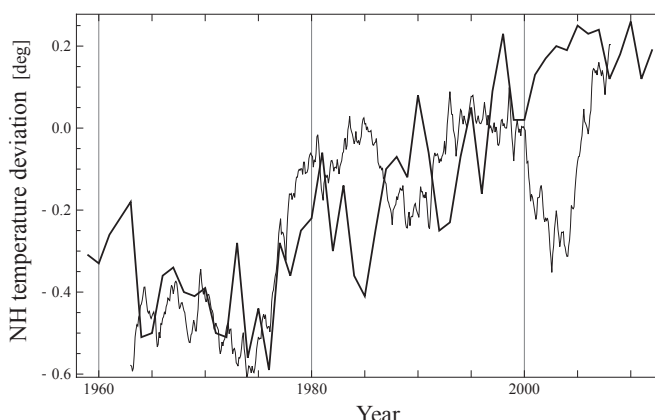
図 10 北半球の温度変動とスケーリングされた振幅の絶対値との比較 (太線が気温の偏差)
