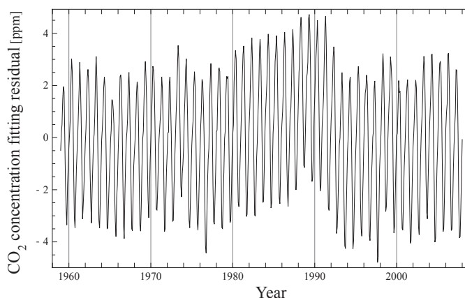
図5 フィッティング後の残差
