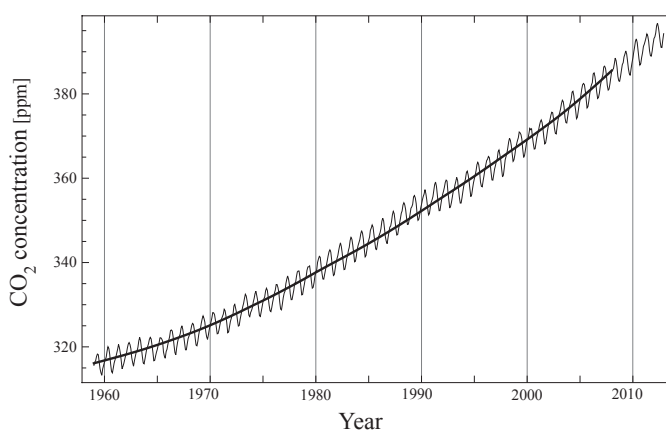
図4 化石燃料燃焼に由来する大気中に排出された炭酸ガスの積算量と Mauna Loa で測定された濃度のフィッティング結果（太線が積算量でフィッティングした結果）
