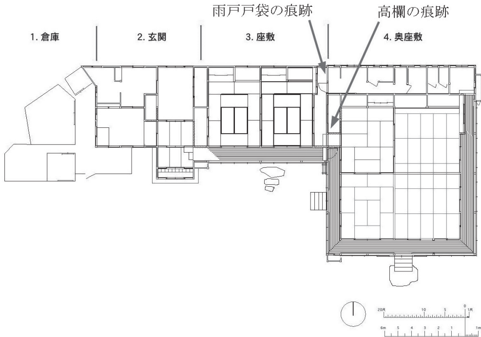
図8：あしべ屋妹背別荘平面図
