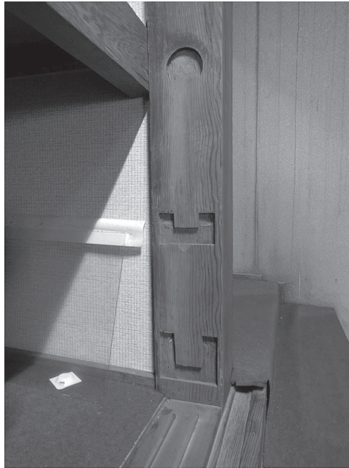
図9：押し入れに残る高欄の痕跡
