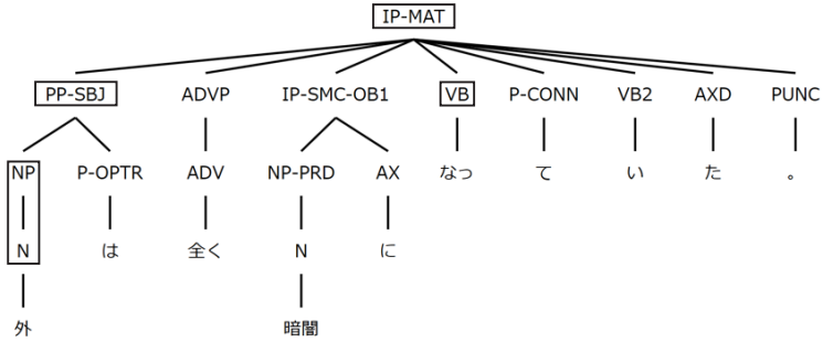
図2 主節動詞述語と主語名詞の例
