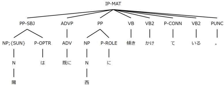
図1 KTBの統語構造
