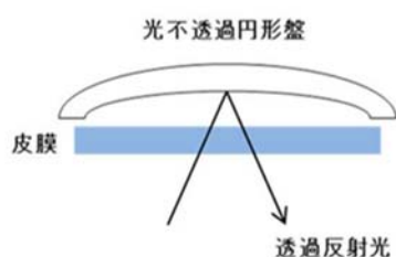
図 2. ゼラチンシートの NIR 測定方法
